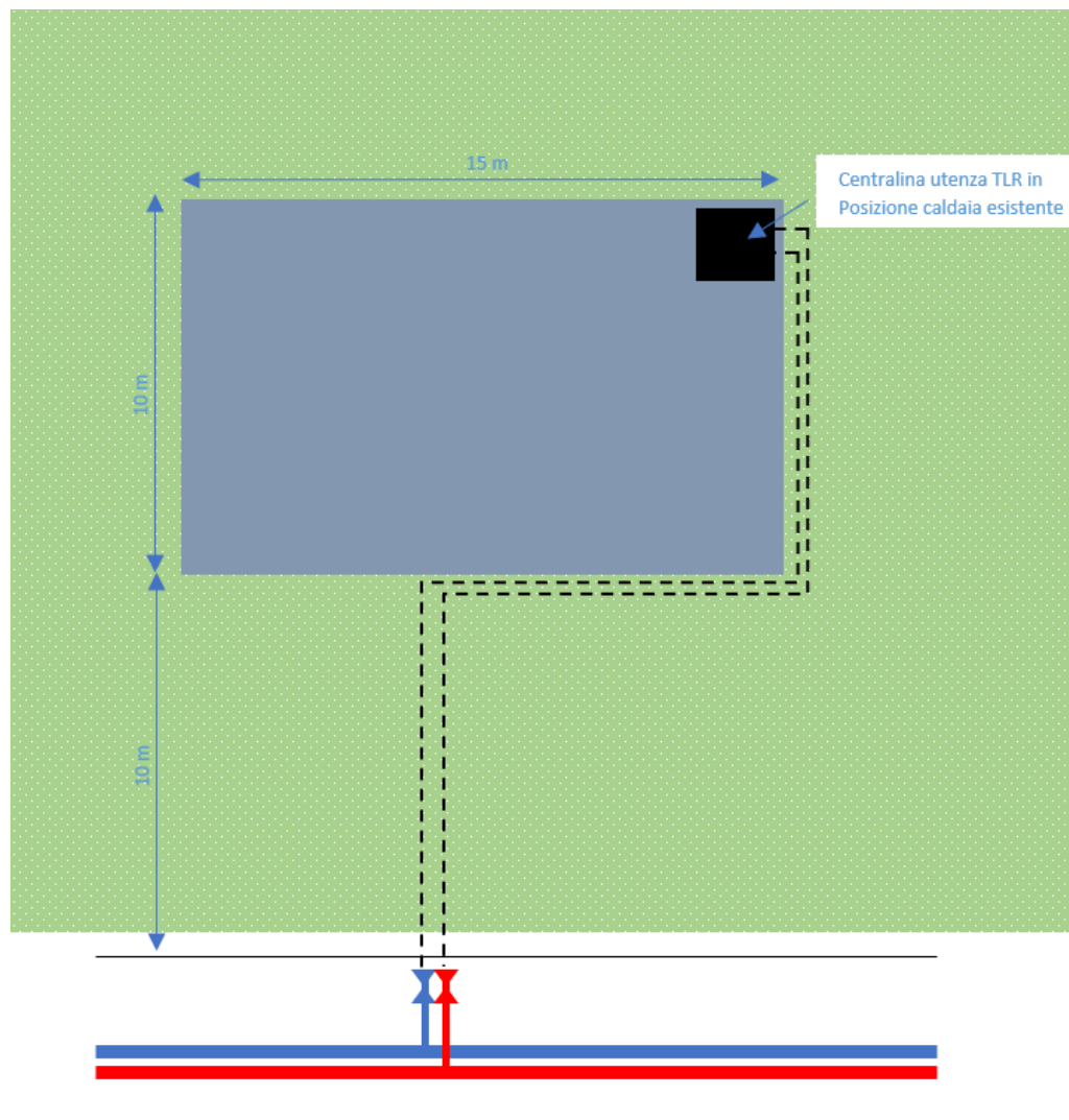
Figura 4 - Planimetria semplificata tipico 4
