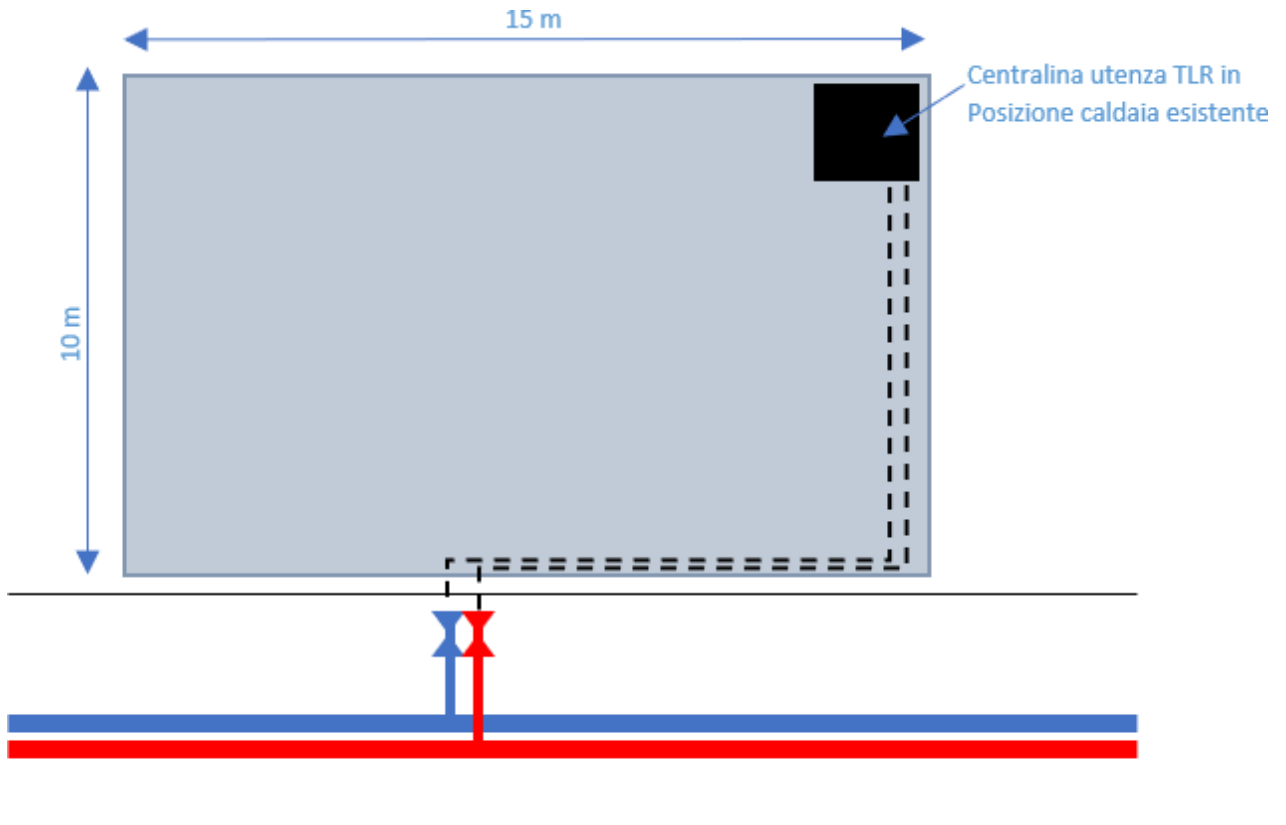
Figura 2 - Planimetria semplificata tipico 2
