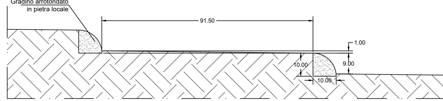
Sezione FF - Scala 1:10
