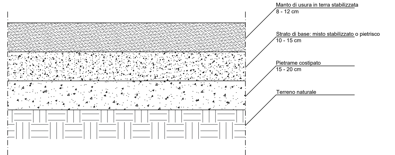
4. Particolare pavimentazione area scala
