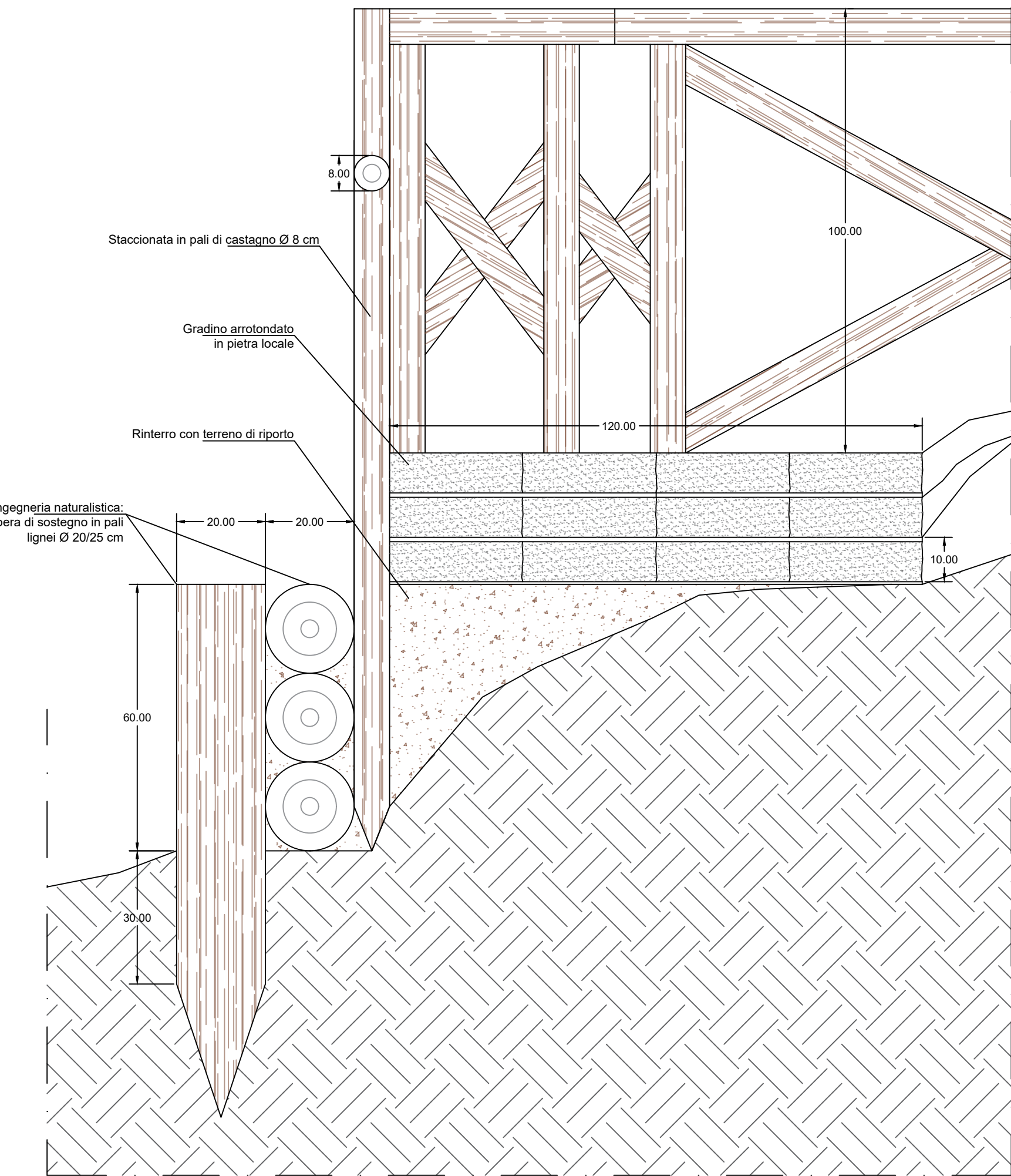
Sezione EE - Scala 1:10
