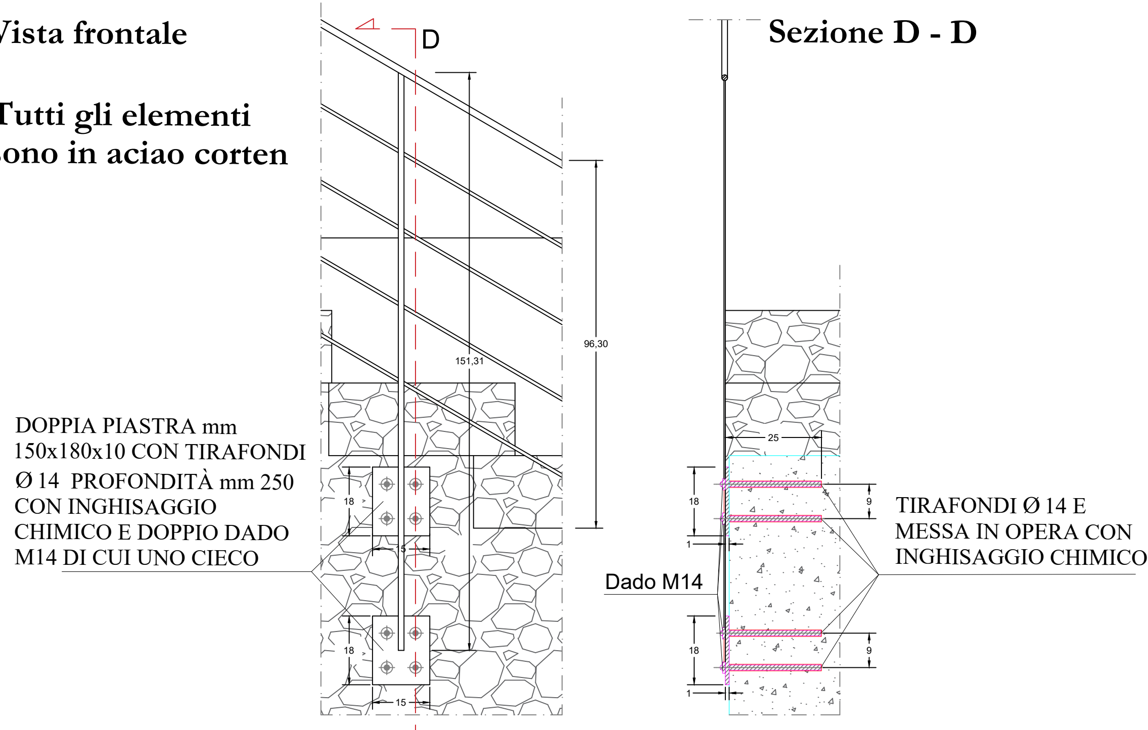
3. Particolare rivestimento muro
